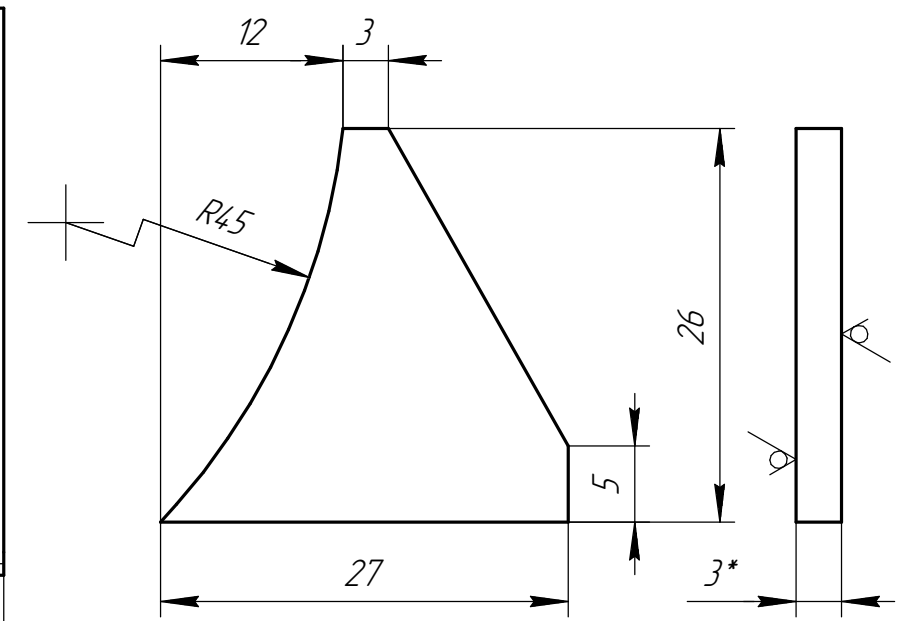
Дет. поз. 5 (2:1)
