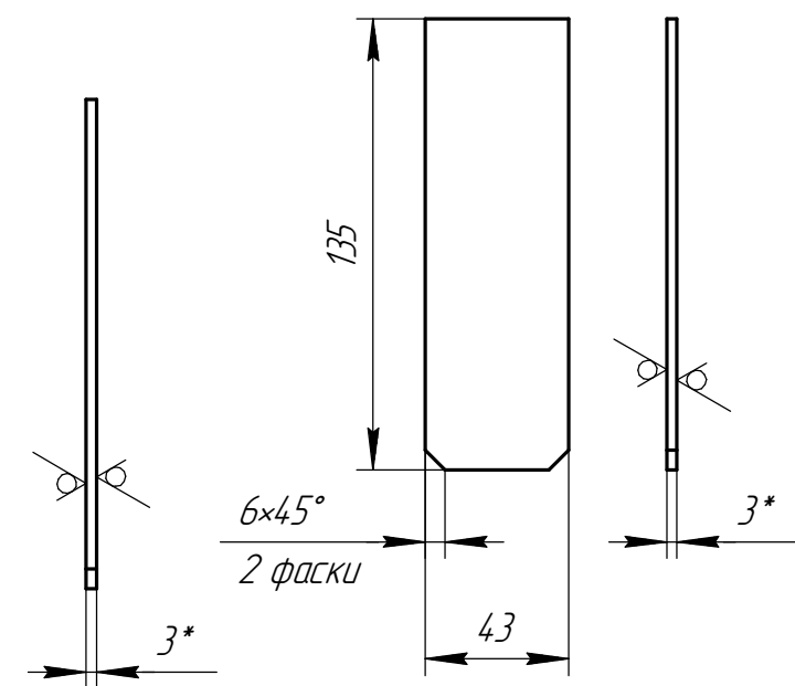
Дет. поз. 4 (1:2,5)
