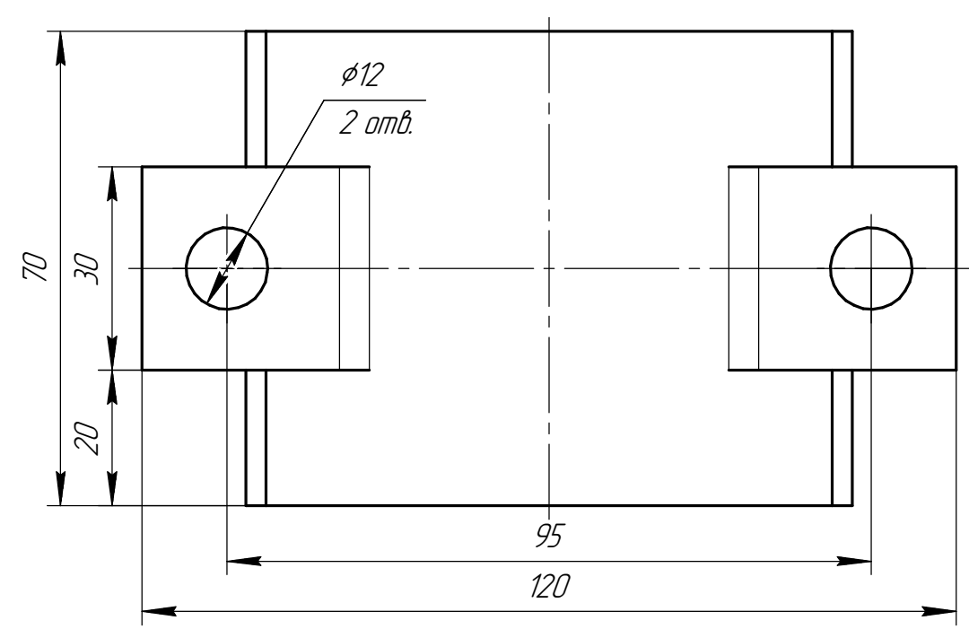
Дет. поз. 4 (1:2,5)
