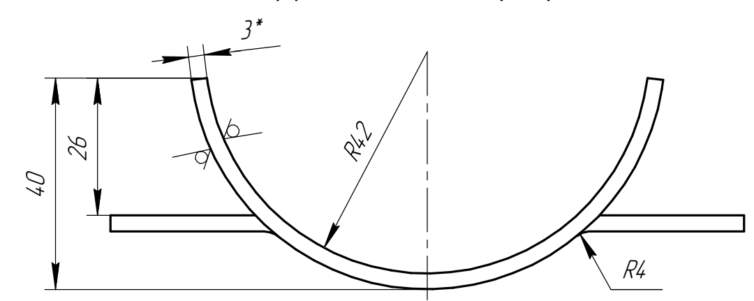
Дет. поз. 2 (1:1)
