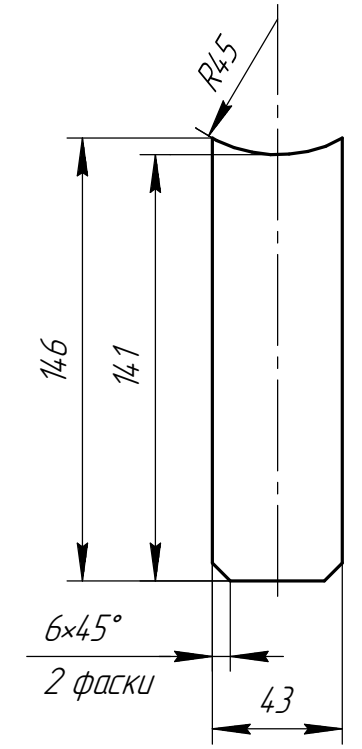
Дет. поз. 3 (1:2,5)
