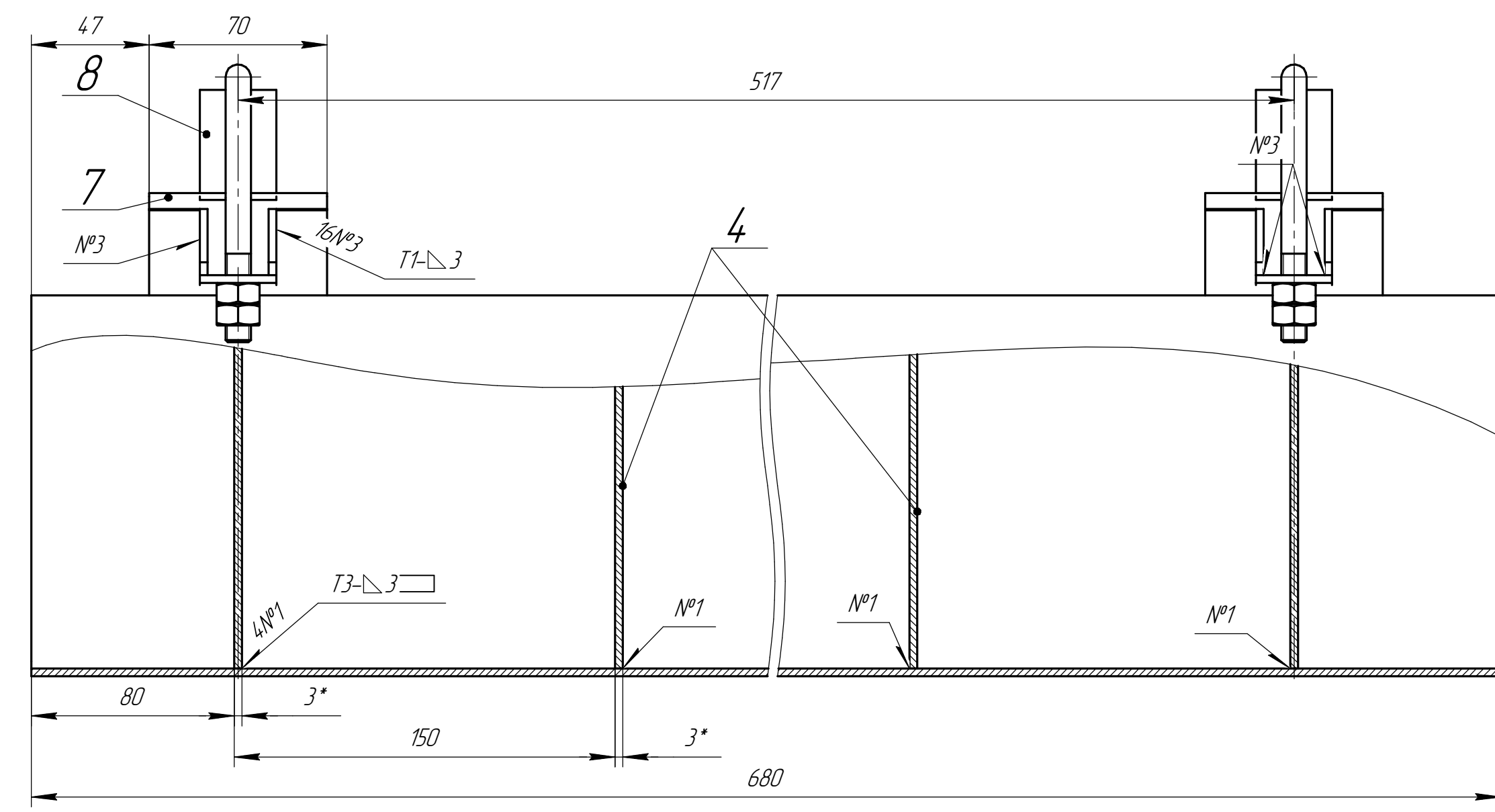
Дет. поз. 2 (1:1)
